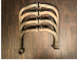
Abgaskrümmer (exhaust manifold)
